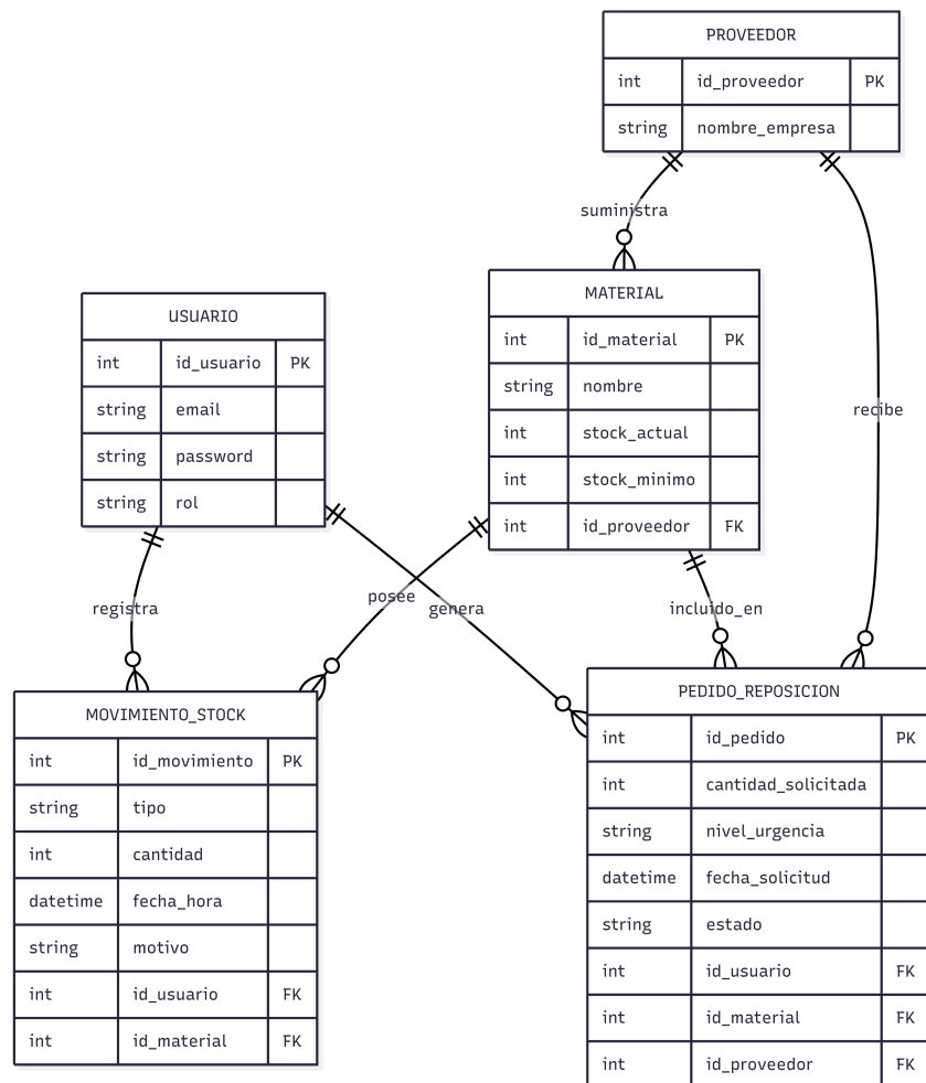
Figura 1: Diagrama Entidad-Relación generado para StockManager
